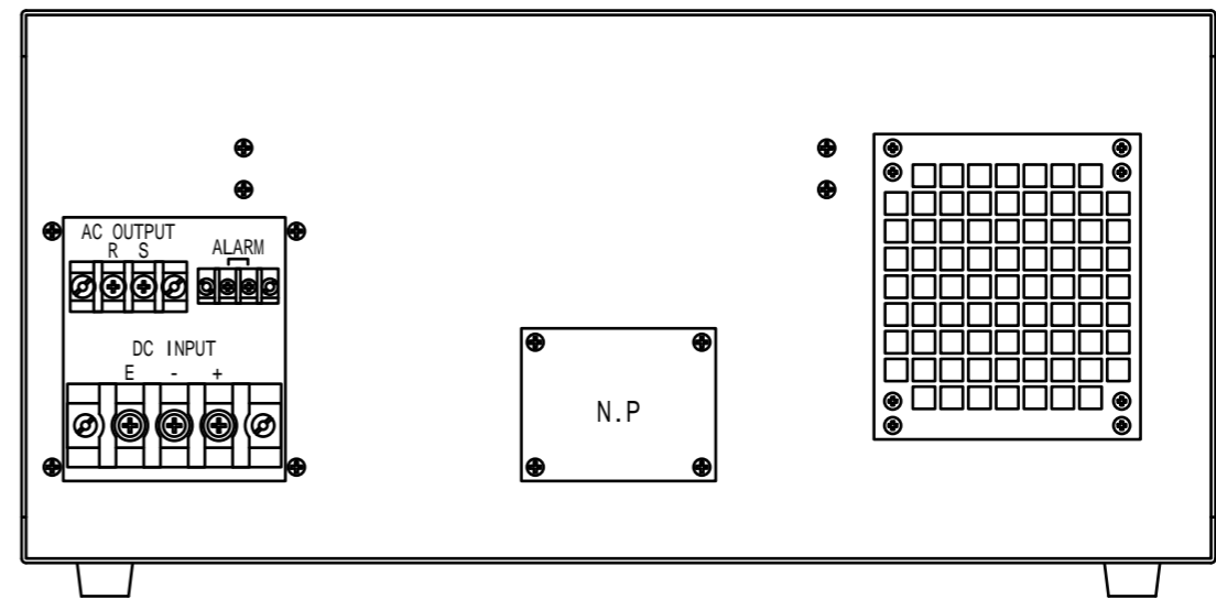
-背面図-
