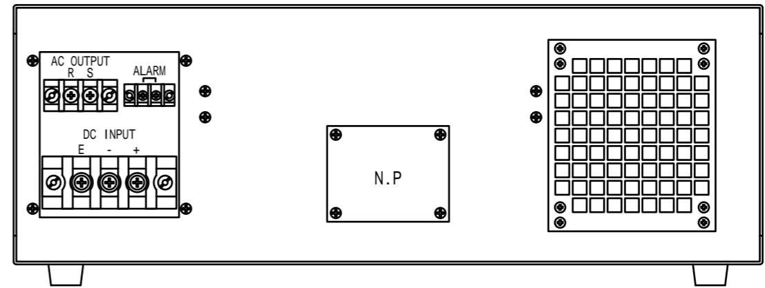
-背面図-
