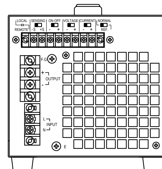
-背面図-
