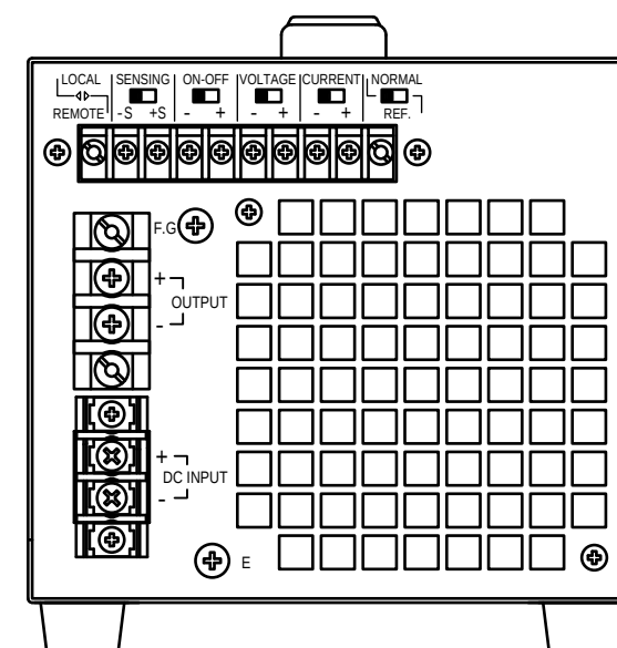
-背面図-
