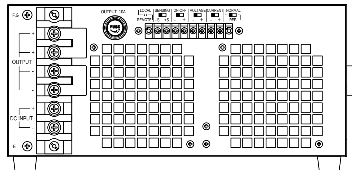
-背面図-
