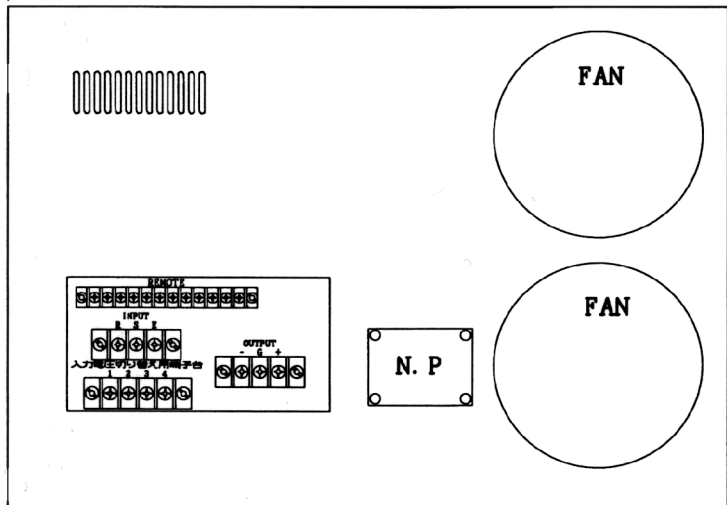
背面図
