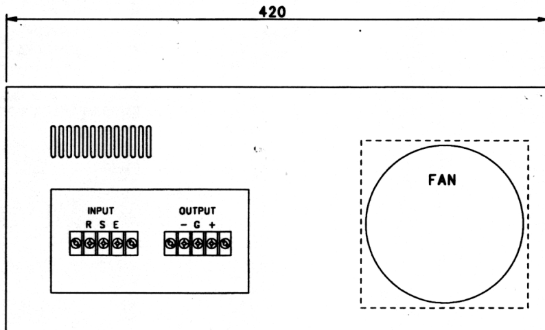
背面図
