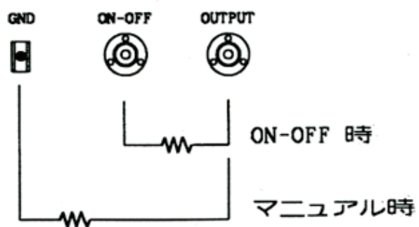
接続図
