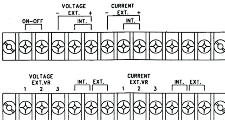
リモート端子詳細図
